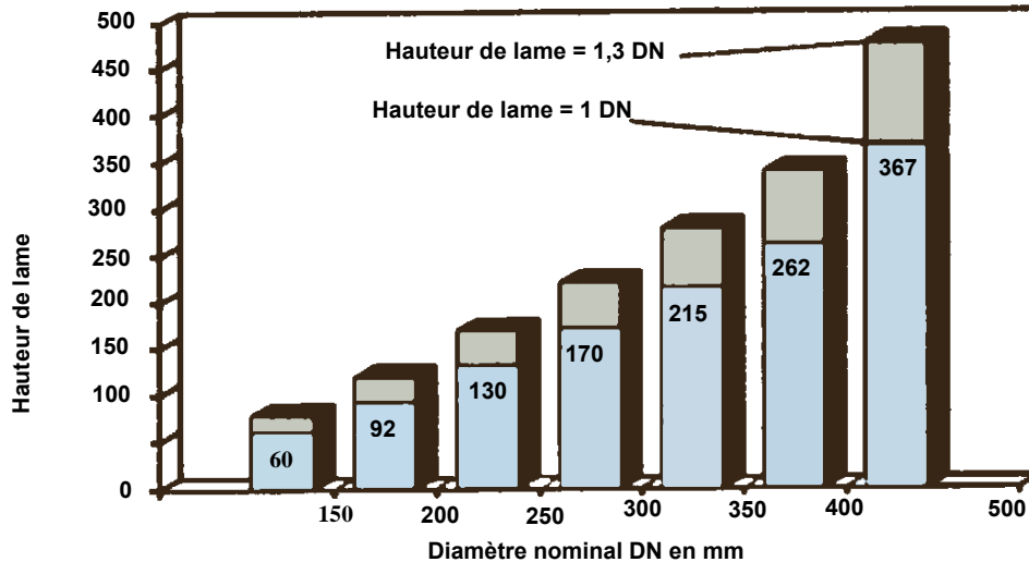
Graphique 5: Domaine d'application du clapet sur seuil HYDROVEX® LCV
