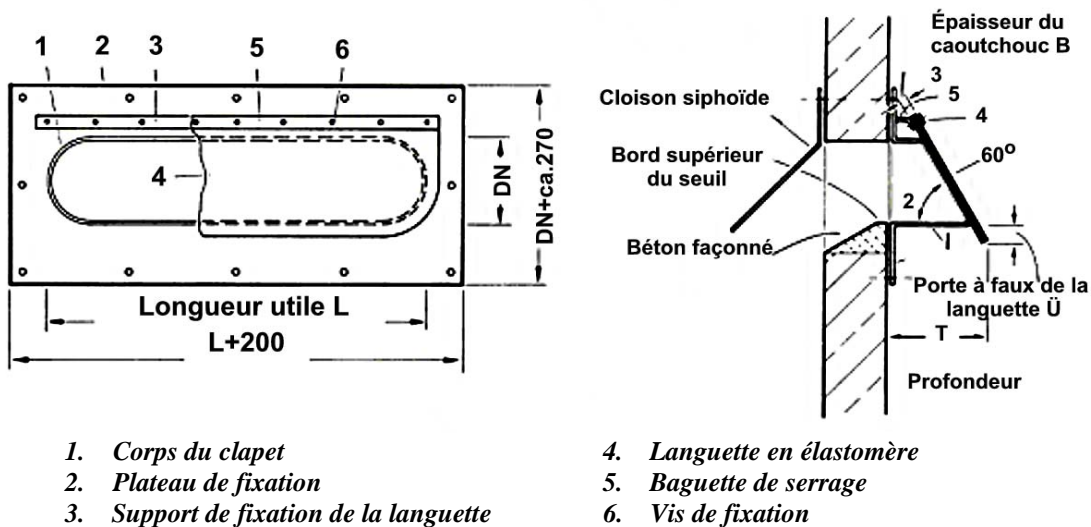
Schéma 2 : Principales pièces du clapet sur seuil HYDROVEX® LCV
