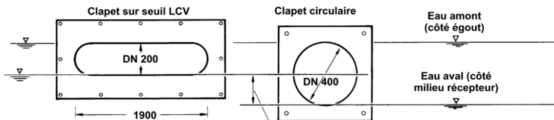
Schéma 1 : Comparaison entre le clapet sur seuil HYDROVEX® LCV et le clapet circulaire.
