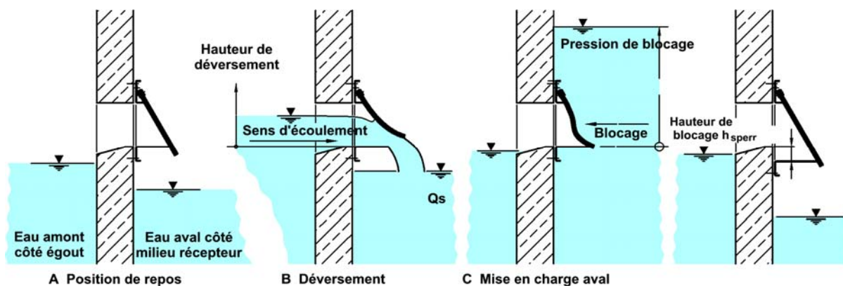
Schéma 3: Fonctionnement du clapet sur seuil HYDROVEX® LCV
