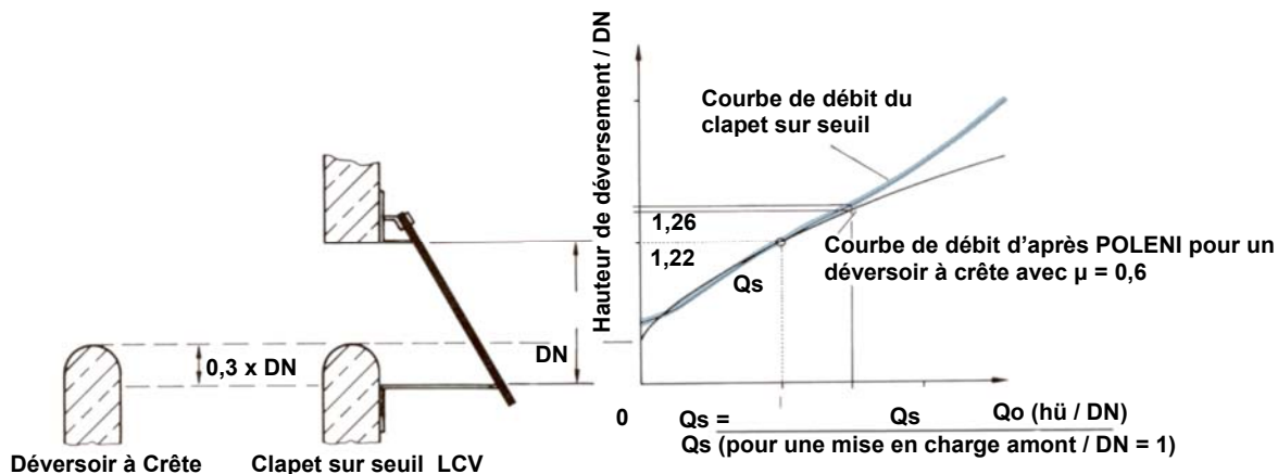
Schéma 4 : Courbes de débit sans dimensions
